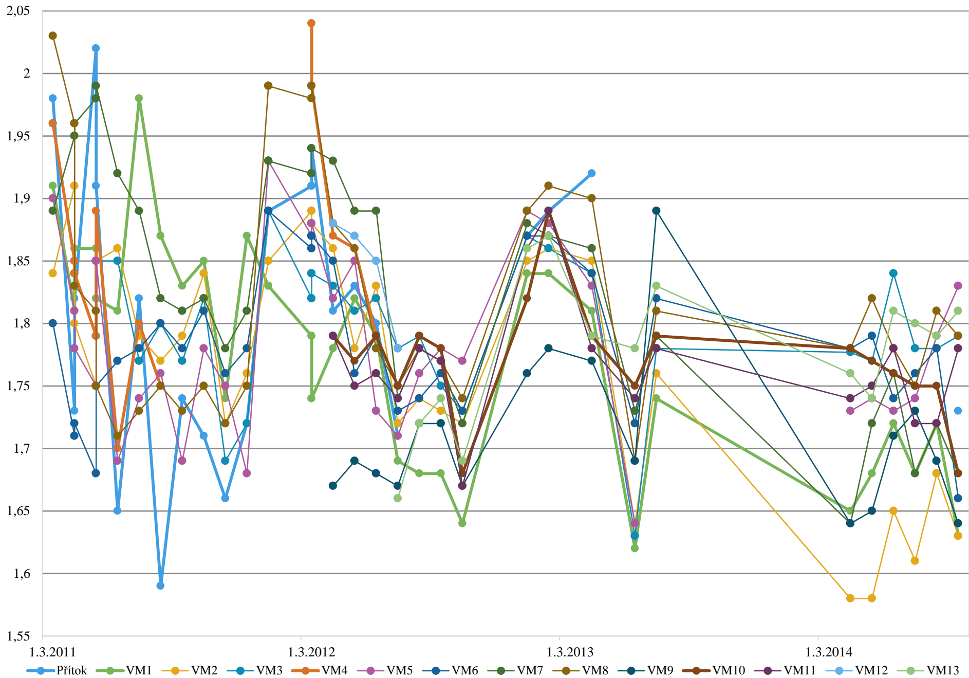
Saprobni index v letech 2011 až 2014 na 14 hodnocených profilech
